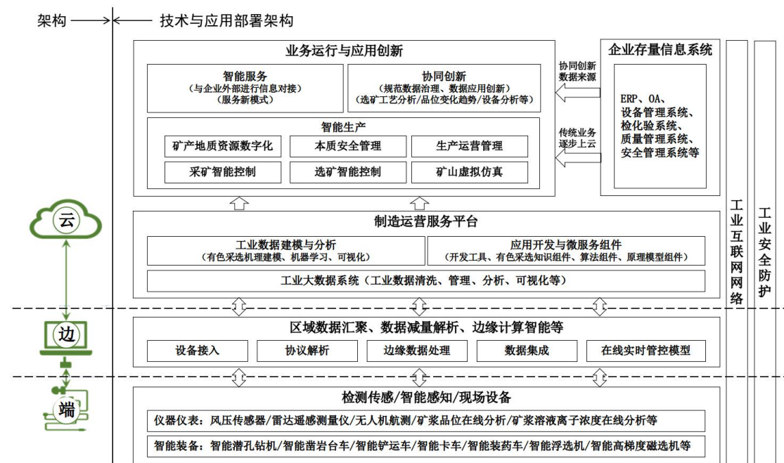
图 1 有色金属智能矿山参考架构图
